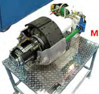
MEGCUT-CHAMBER
